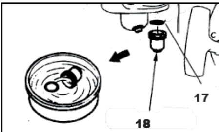
Absatzbecher reinigen
