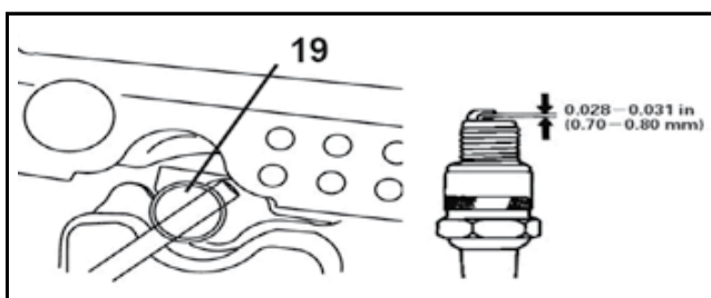
Zündkerze wechseln
