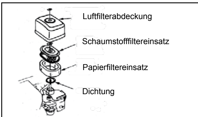
Luftfilter reinigen
