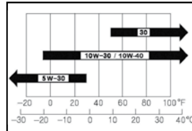
Motorenöl
