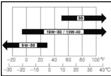
Motorenöl
